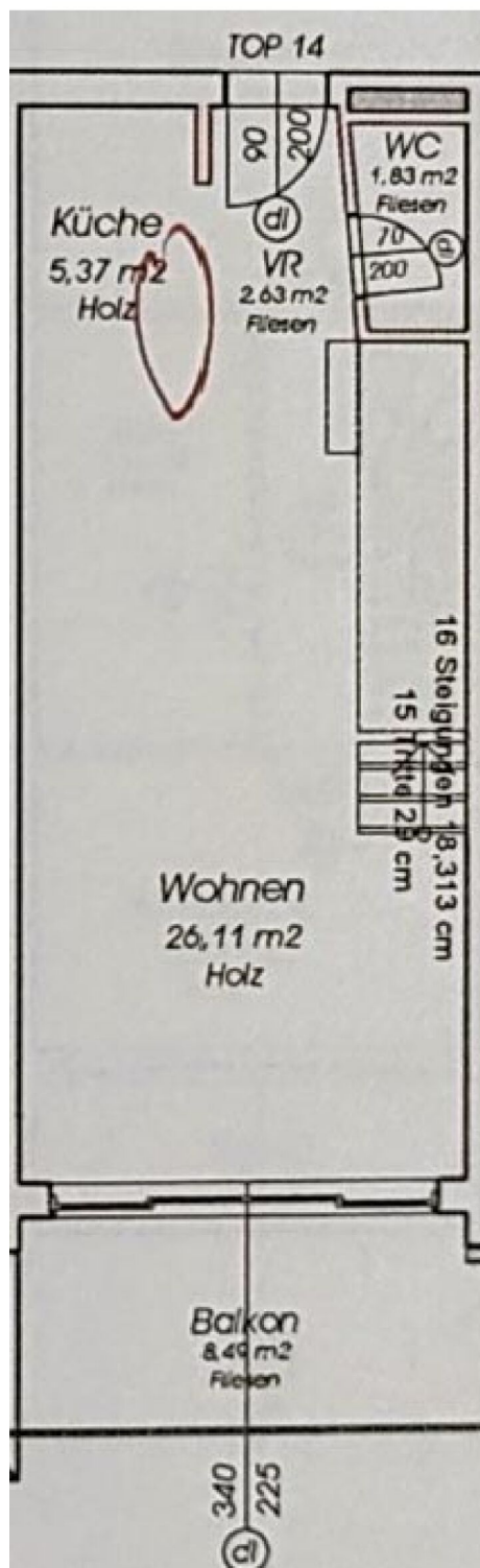
OG2
